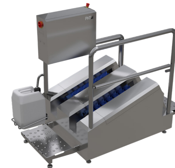
Bild.55 Durchlaufreinigungsmaschine für Stiefel und Schäfte Typ 23835
