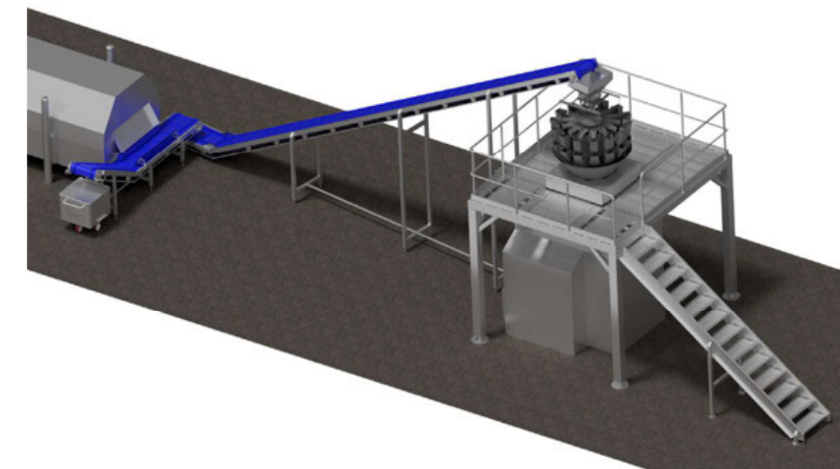
Bild.43 Förderanlage mit Podest
