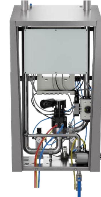
Bild.90 Automatanlage, geöffnet
