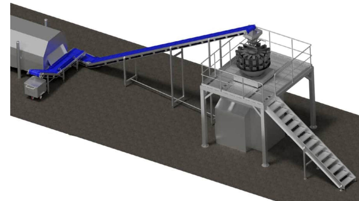
Bild.33 Förderanlage mit Podest
