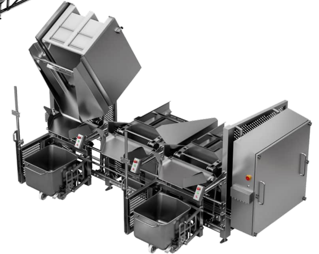
Bild.45 Chargieranlage 800
