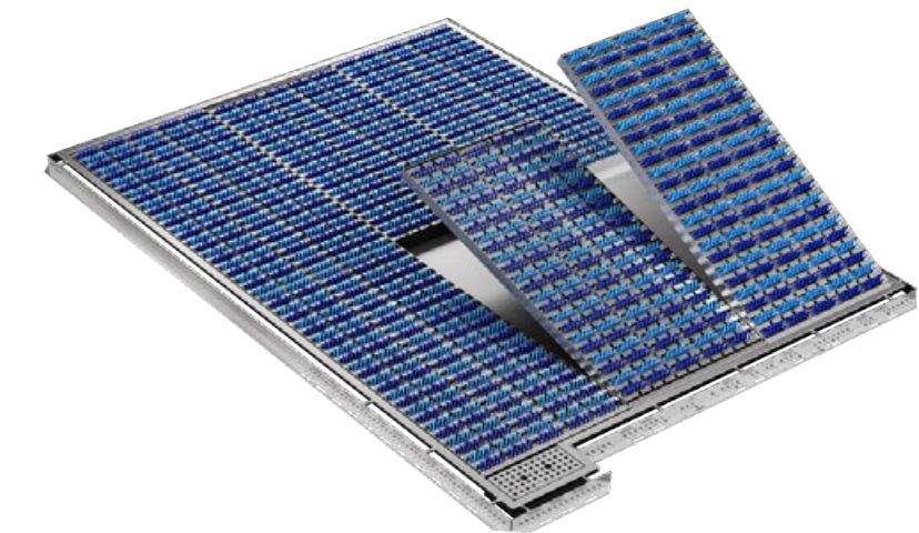
Bild.100 Hygienic Floor System mit geöffneten Kassetten
