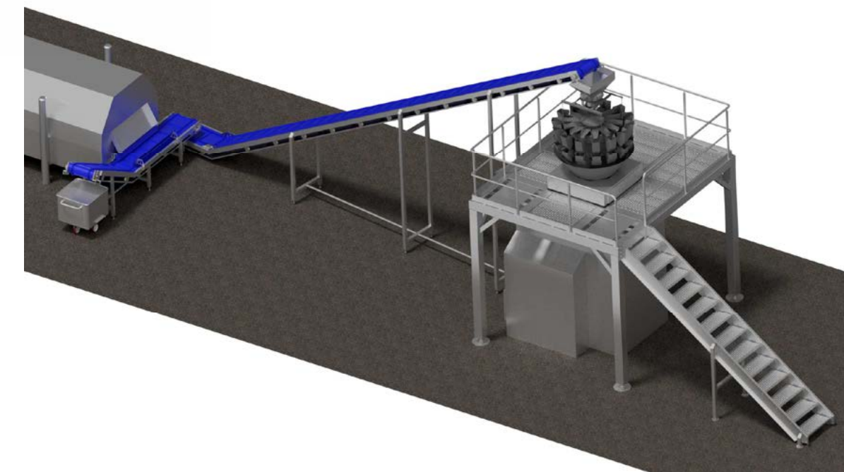
Bild.33 Förderanlage mit Podest
